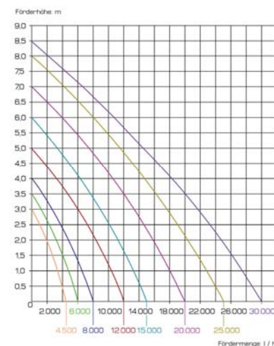
Pumpenkennlinien FIAP Aqua Active Profi
